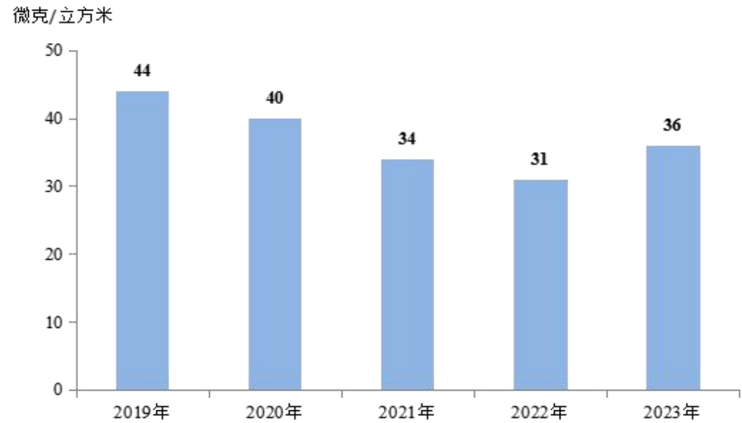
图 8 2019 年—2023 年细颗粒物 (PM2.5) 年均浓度
