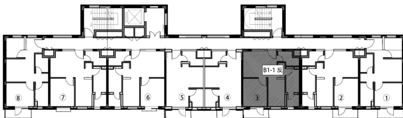
( 四区 2、4 号楼标准层偶数层层户型平面布局图 )
