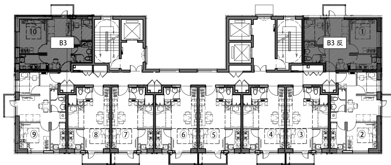
( 四区 1 号楼标准层层户型平面布局图 )
