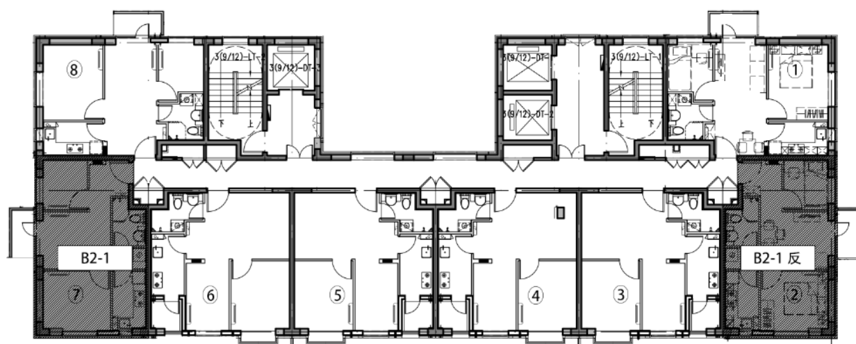
( 三区 4 号楼标准层层户型平面布局图 )
