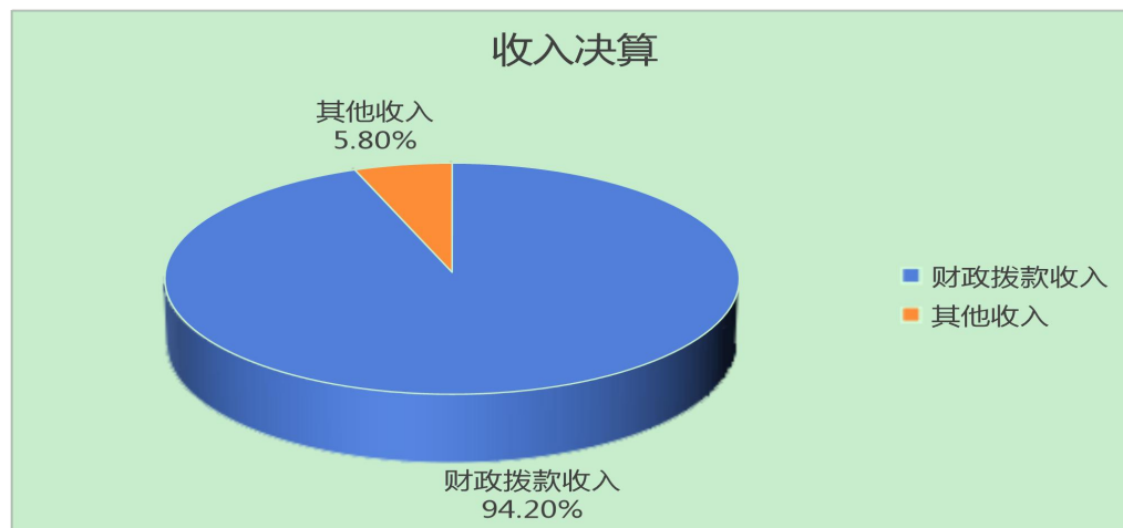
图 1：收入决算
